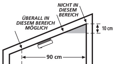
Zeichnung "C"
